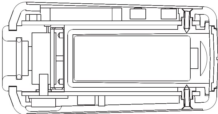
Fig. 3 Costruzione meccanica del calibratore (sezione).
